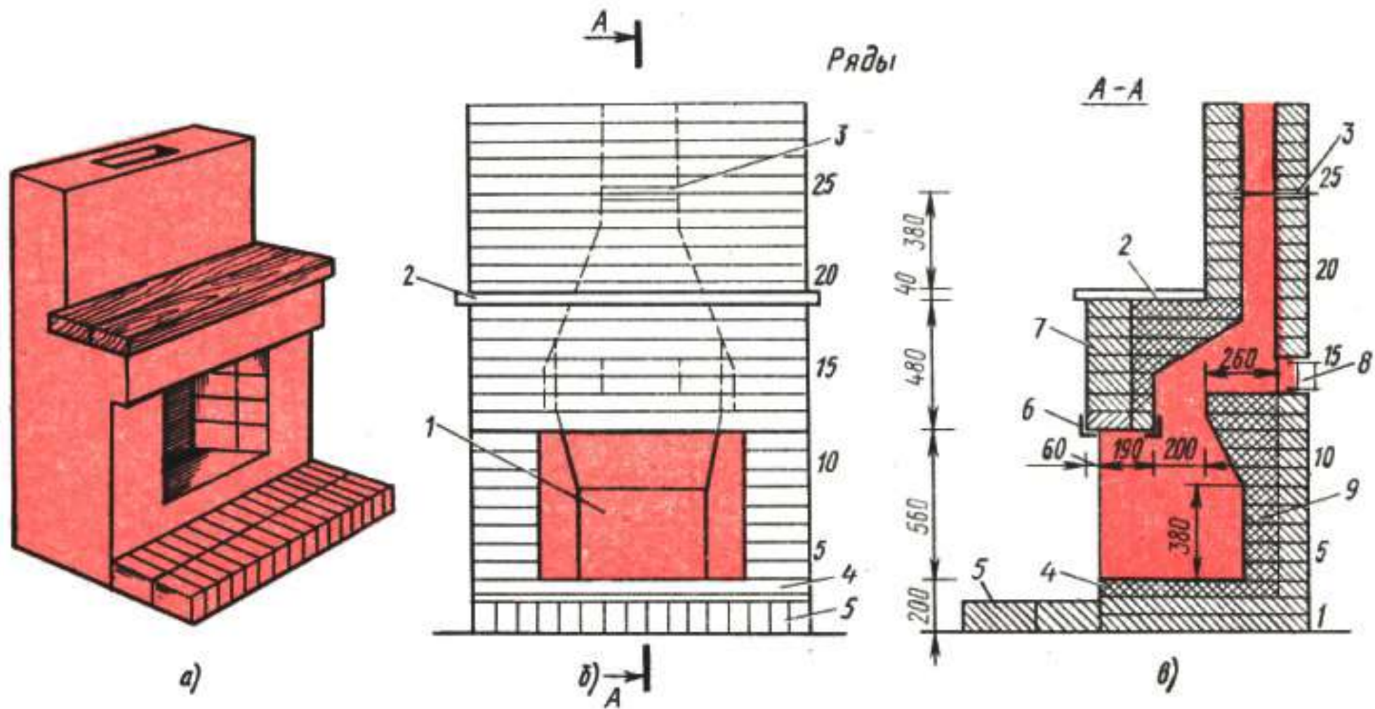
Рис. 102. Камин упрощенной конструкции:
