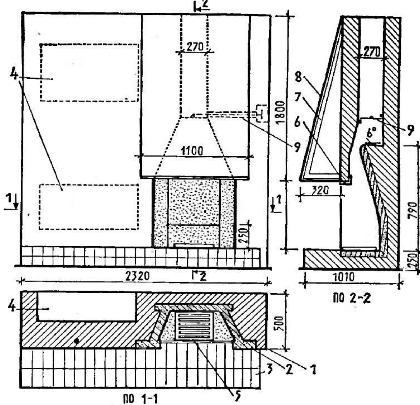
Камин с декоративной стенкой. 1 — кирпичная кладка, 2 — огнеупорный кирпич, 3 — декоративная кладка, 4 — декоративные ниши, 5 — решетка, 6 — металлический уголок, 7 — металлический каркас кожуха, 8 — декоративный кожух (чеканка), 9 — поворотный шибер.
