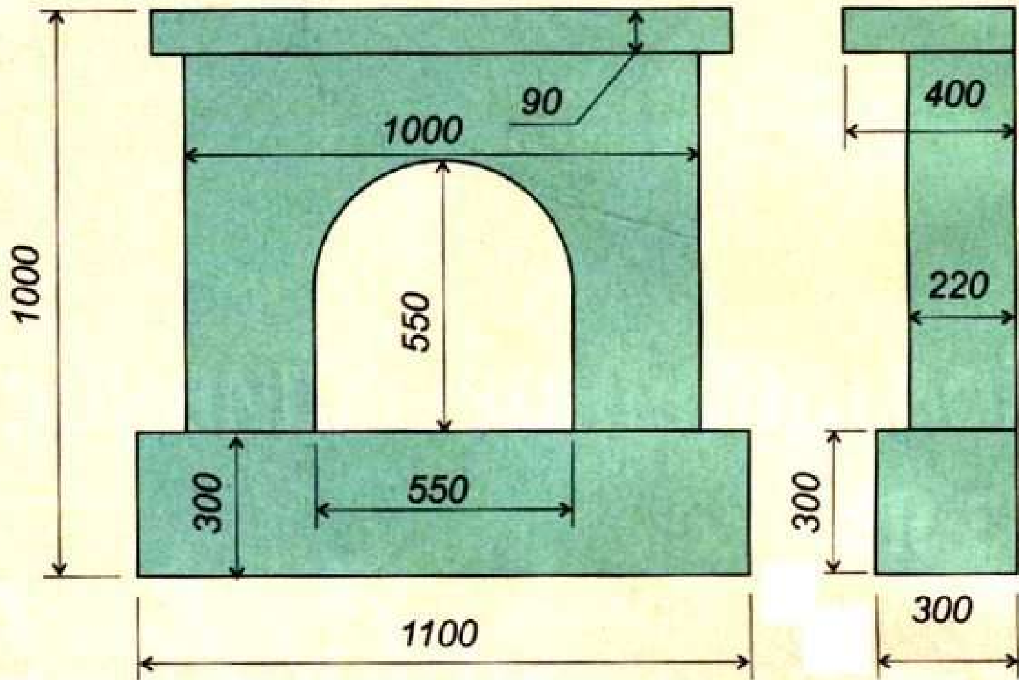
Приблизительные размеры камина
